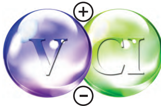
Abb. 2: Schematische Darstellung eines VCI-Moleküls
